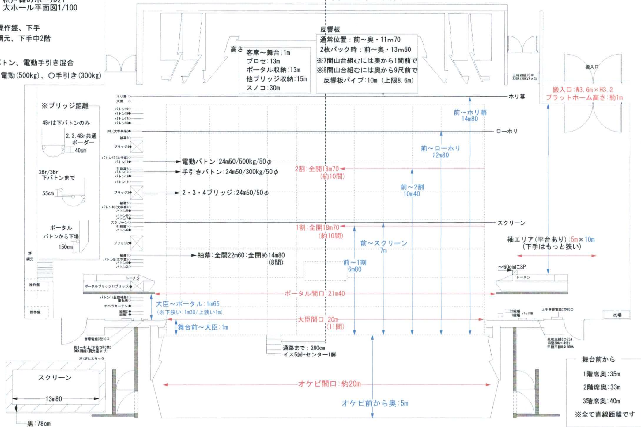
森のホール21：大ホール：舞台基本寸法表
